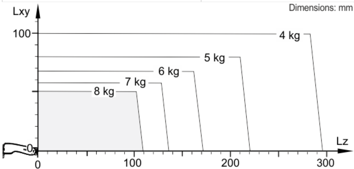
负载能力图，KR 8 R1620 arc HW
